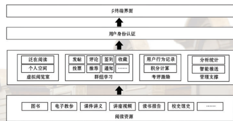
图1 系统框架图
